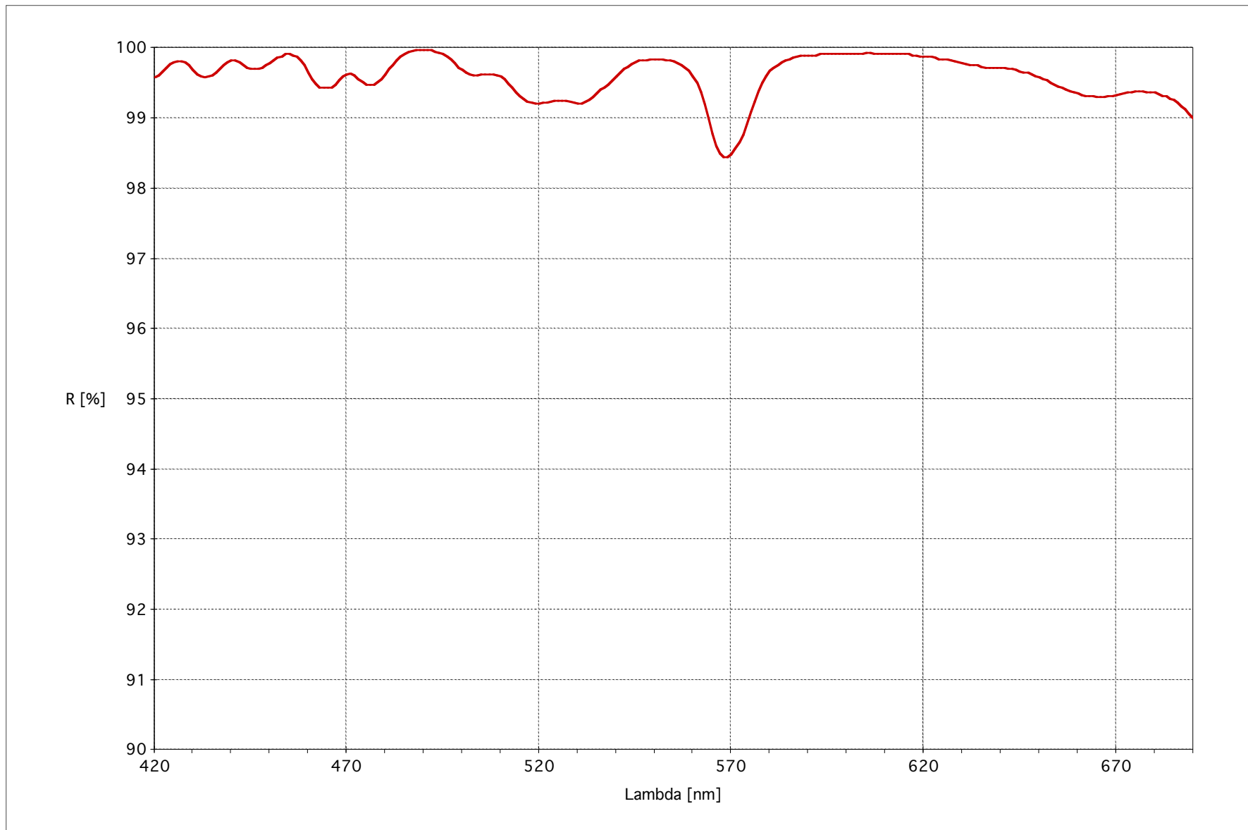
SHR Oberflächenspiegel (Skalierung der Y-Koordinate 90-100% !), 420-690nm
